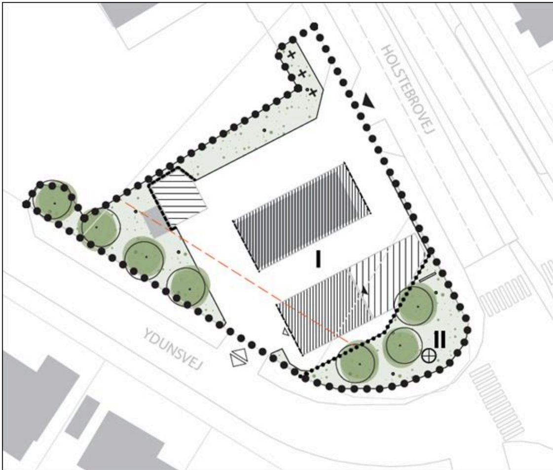
Kortbilag 2. Lokalplankort
