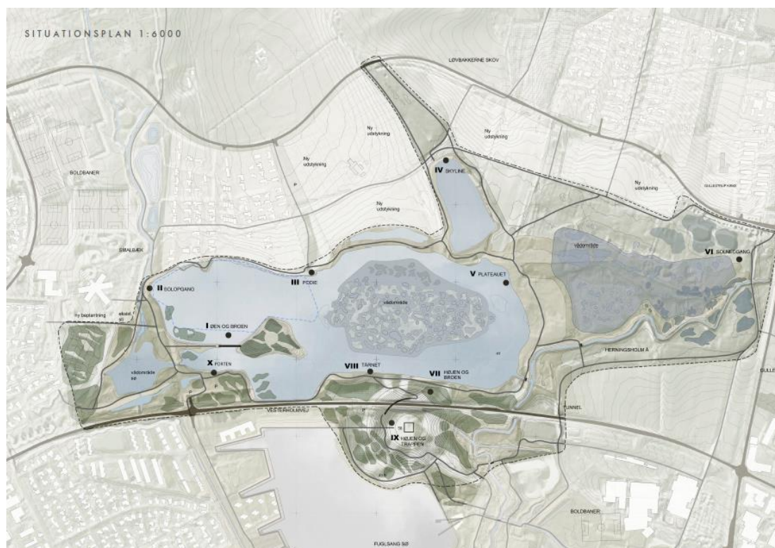
Landskabsplan Holing Sø 1:6.000. Markører I-X vises på illustrationen samt vedhæftede bilag 'Landskabsplan Holing Sø'. Udarbejdet af Tegnestuen DETBLÅ.
